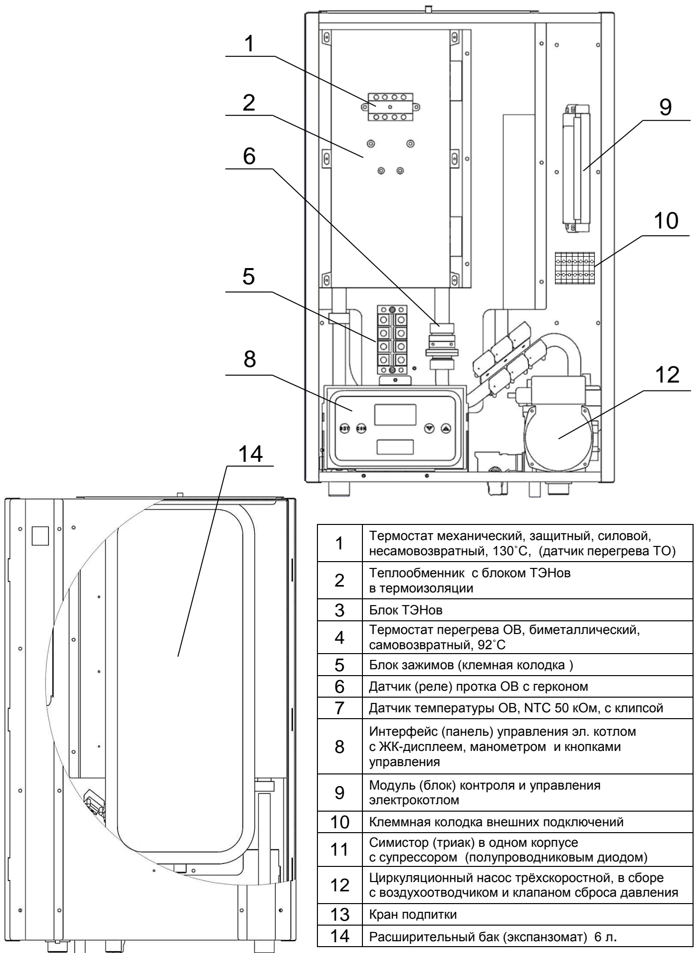
Рис. 2 Внутренне устройство
