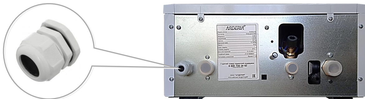
Рис. 13 Кабельный ввод
