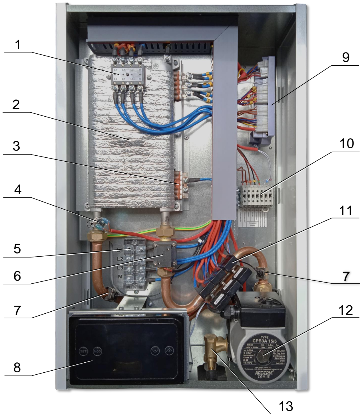
Рис. 1 Общий вид
