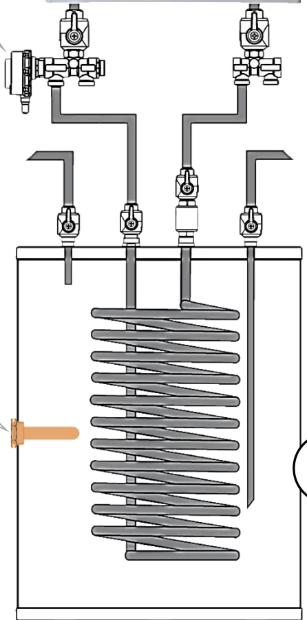
Рис. 22 Принципиальная монтажная схема подключения электрокотла к емкостному водонагревателю косвенного нагрева (бойлеру)
