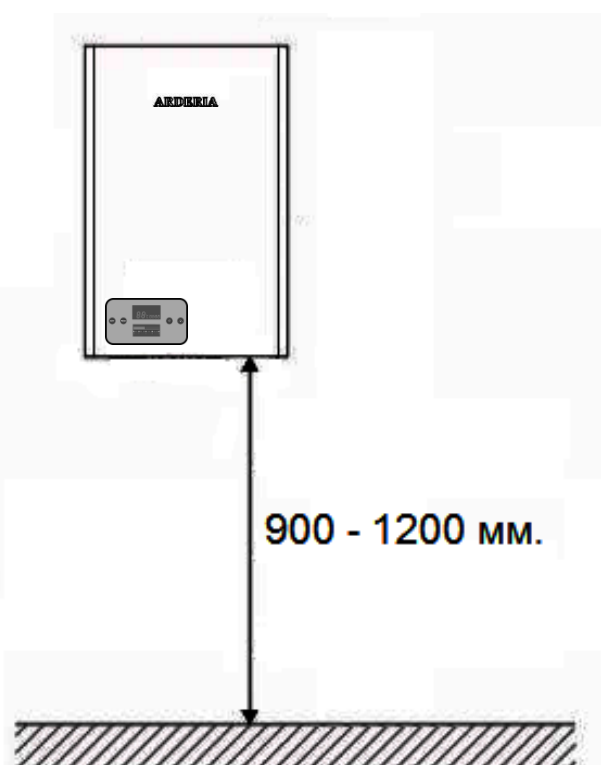
Рис. 10 Монтажные расстояния
